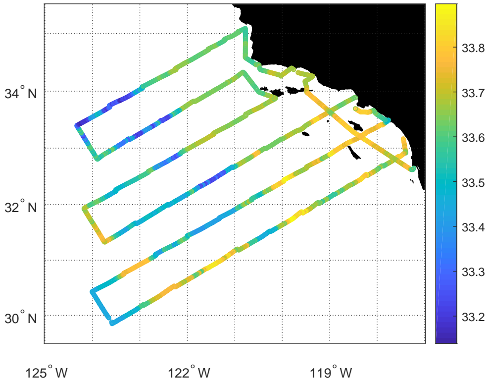
CalCOFI CC1810 - SS Sal
