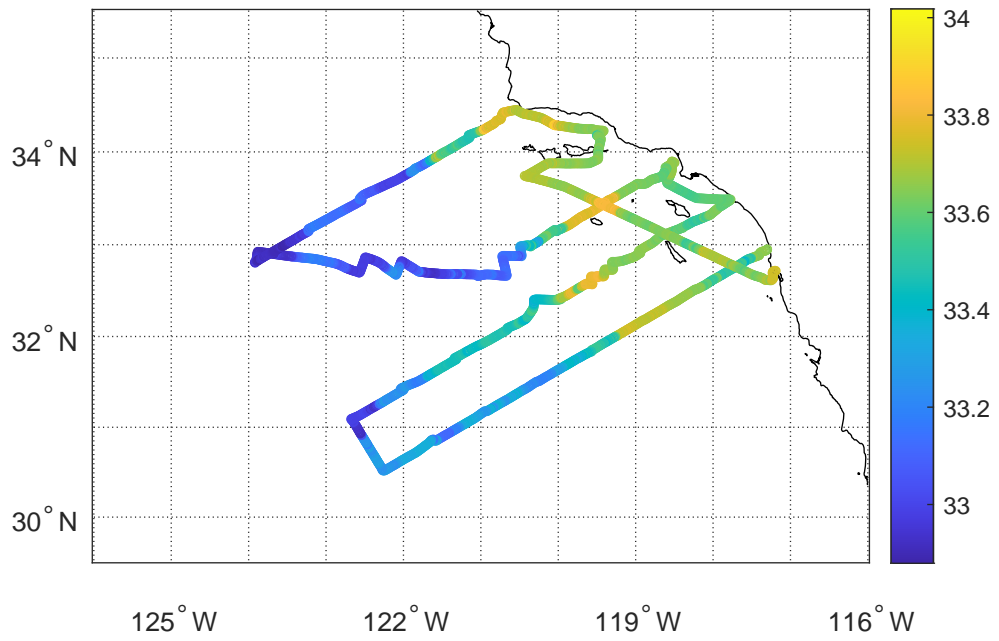
CalCOFI CC2105 - SS Sal
