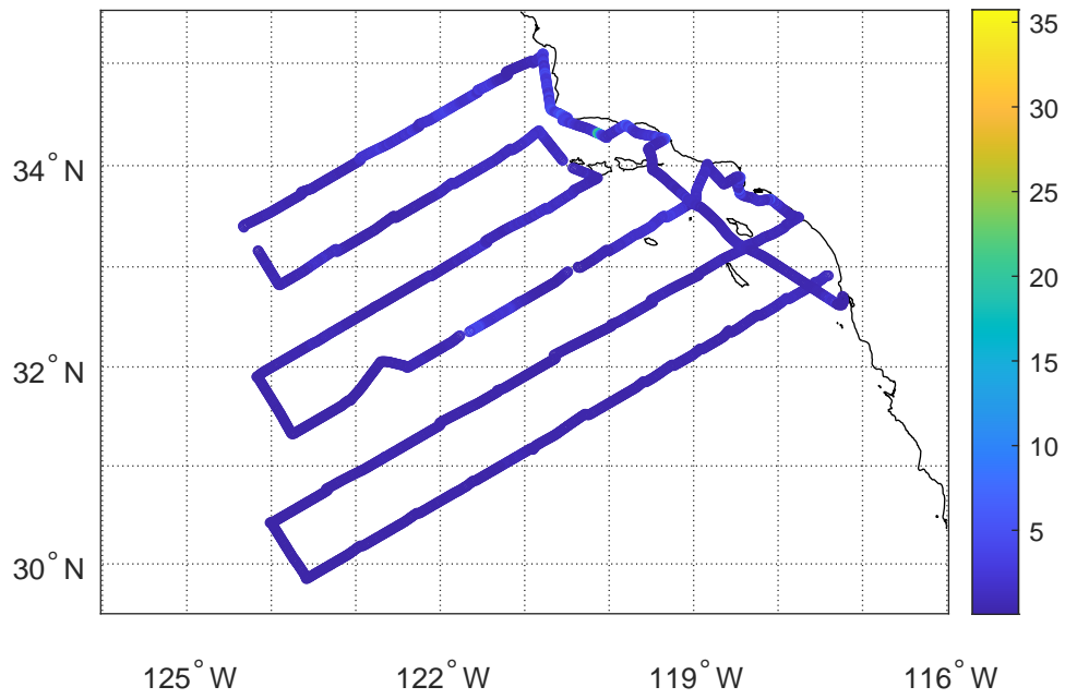
CalCOFI CC2111 - SS Chla
