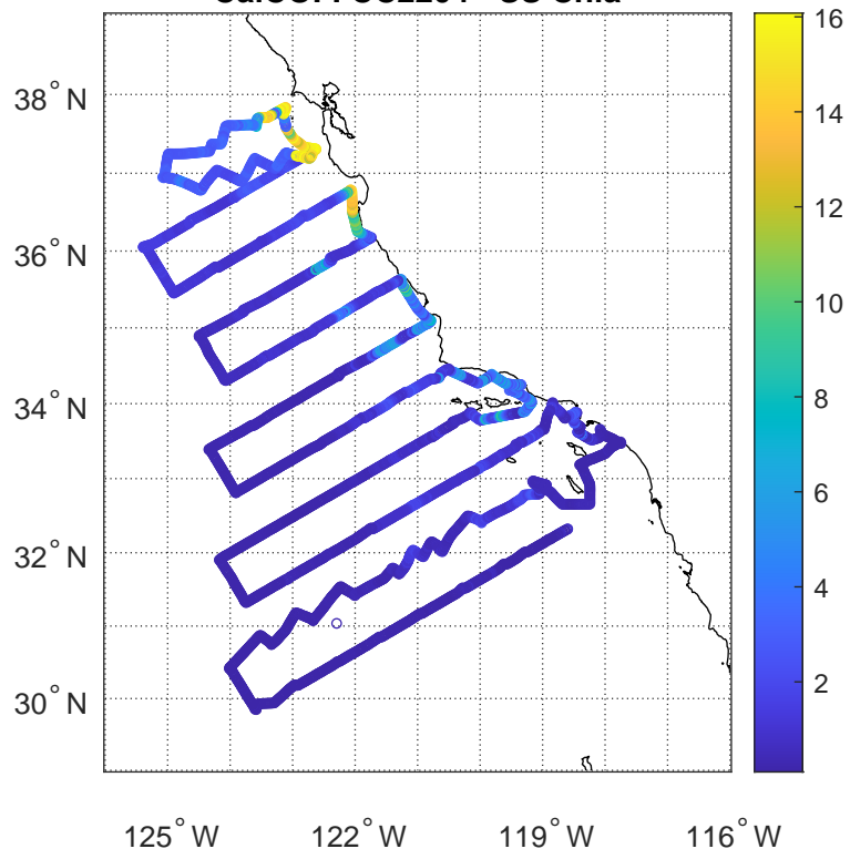
CalCOFI CC2204 - SS Chla
